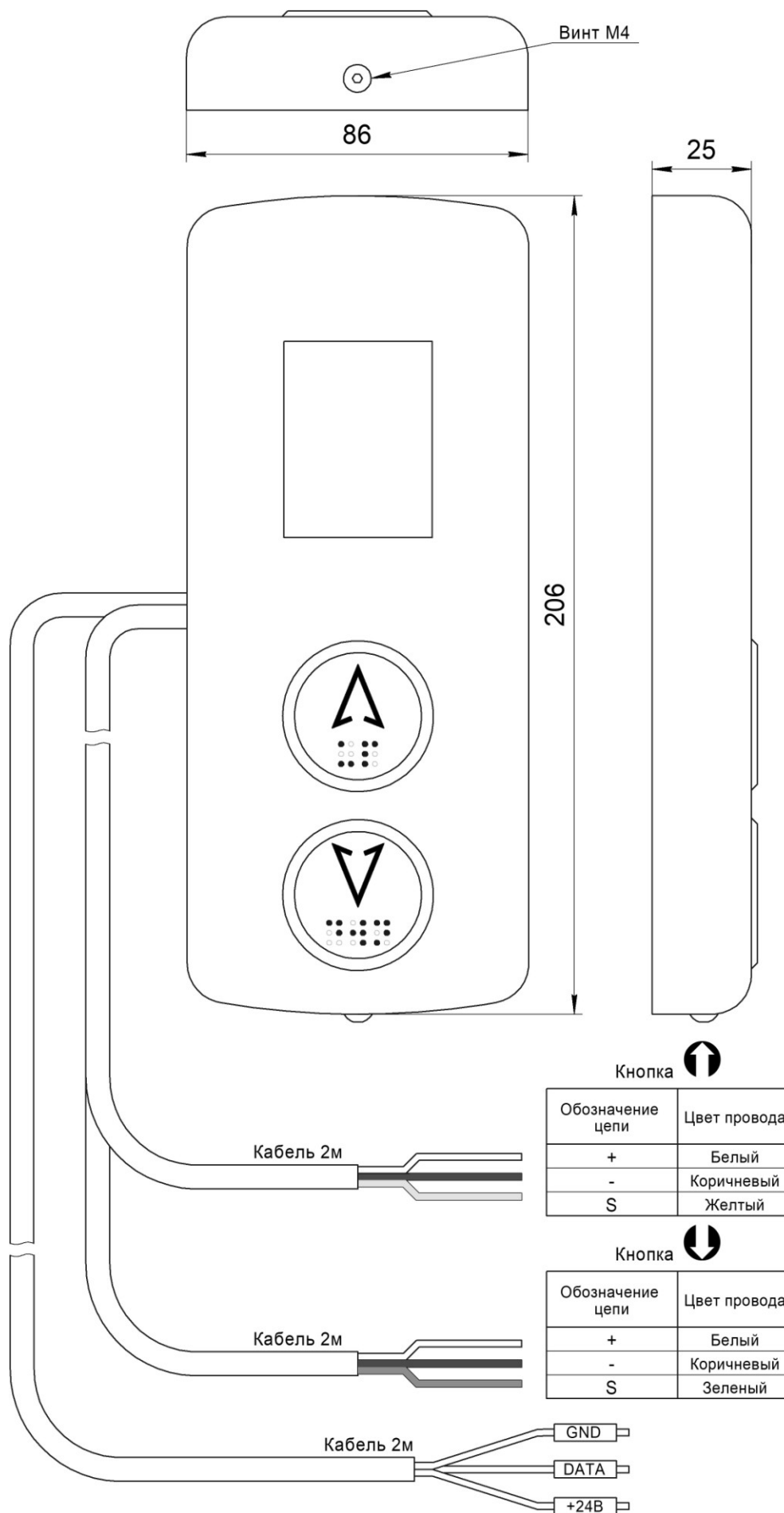
Рис.1 Внешний вид, габаритные и установочные размеры Вызывного поста ВП-2103-1074-08
